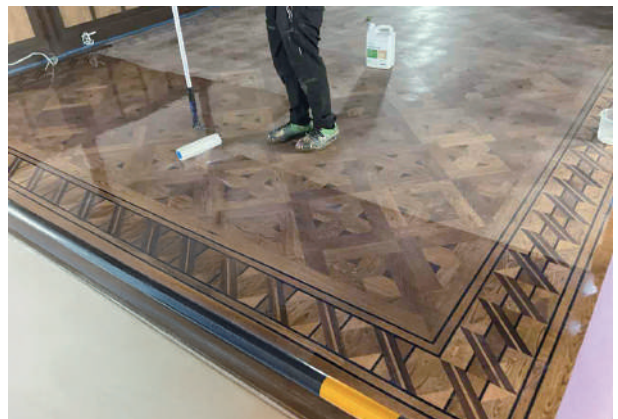
4 寄木上塗りトップコート施工状況
