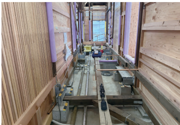
13 廊下1床下配管状況
