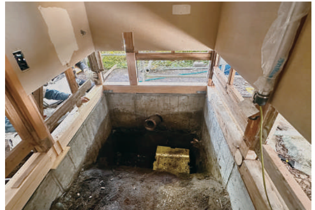
22 別棟トイレ土台入替状況
