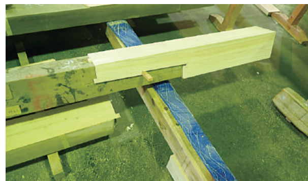
31 柱根接ぎ補修
