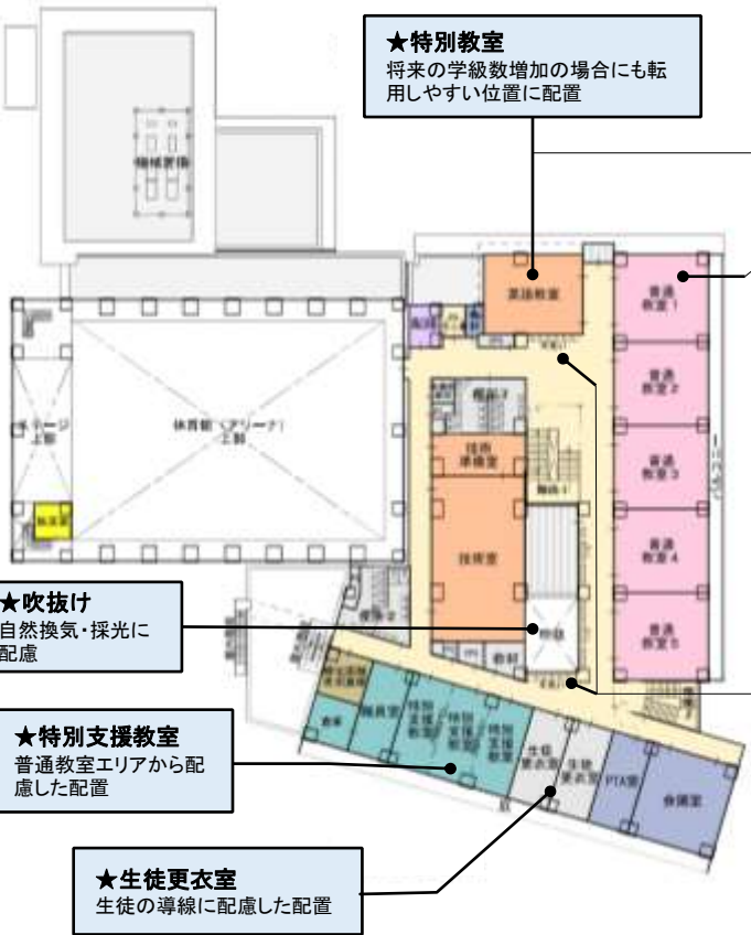
<2階平面図>
