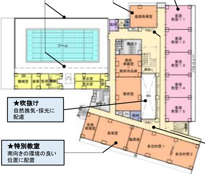
<4階平面図>
