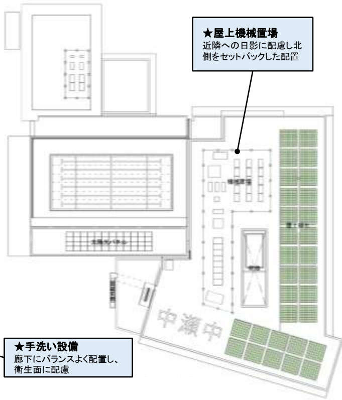
<R階平面図>
