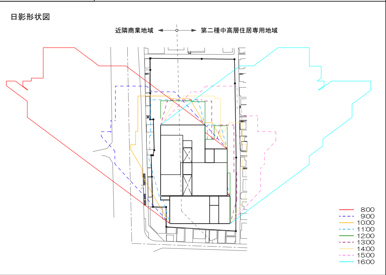
B-1. 南西側配置案 ※新規作成案
