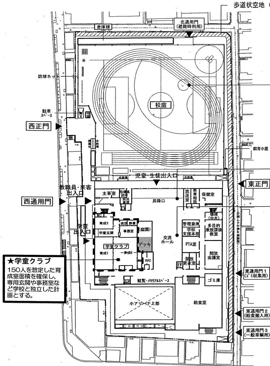
1 F ・ 配置図
