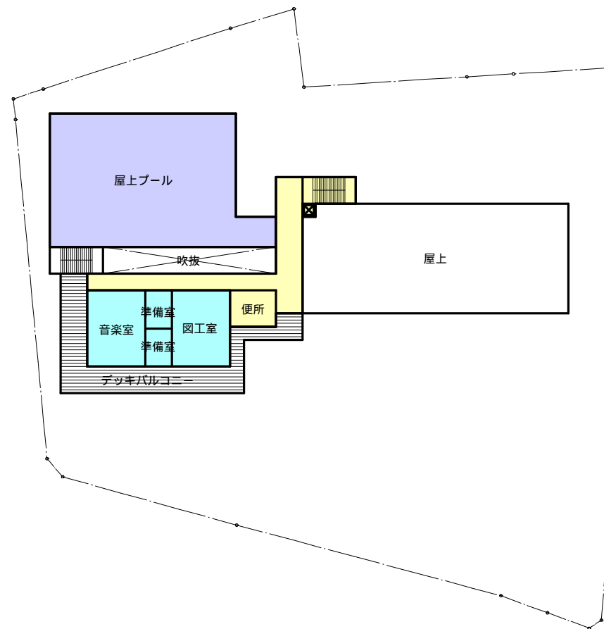
4階平面図
