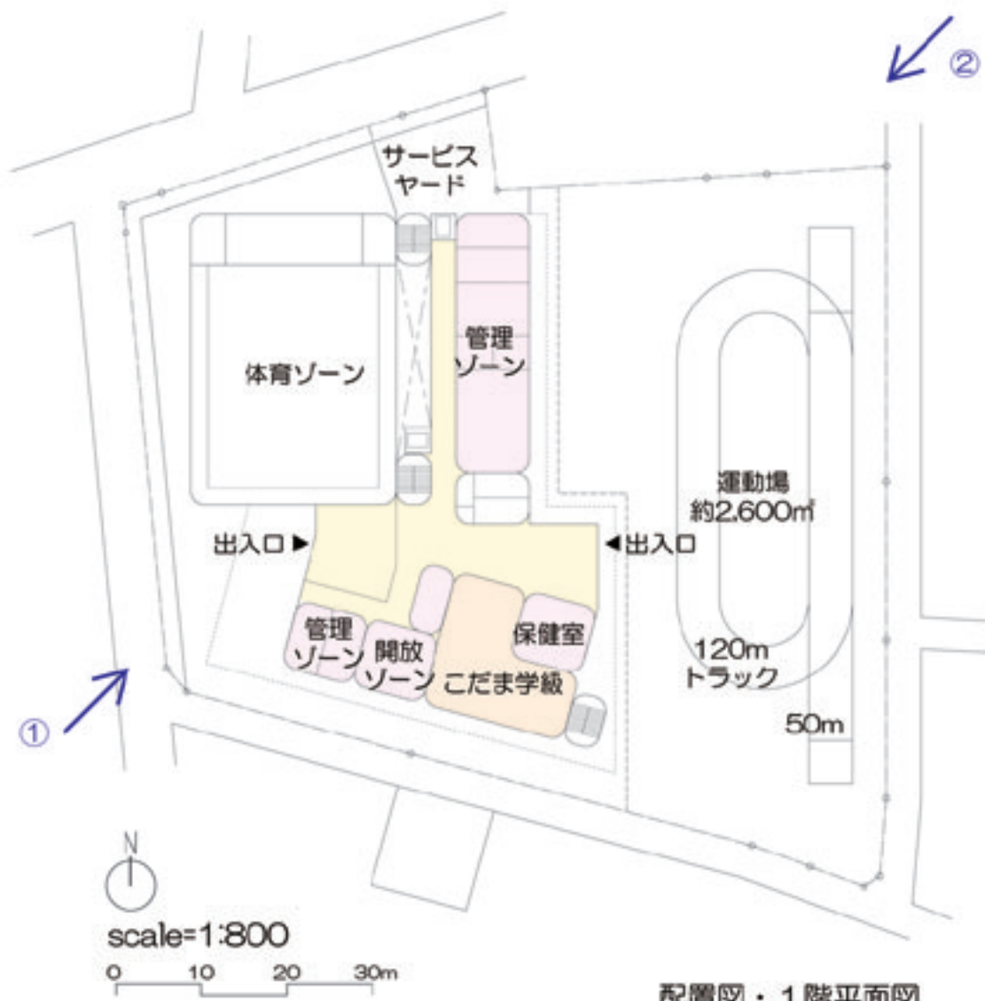
配置図・1階平面図
