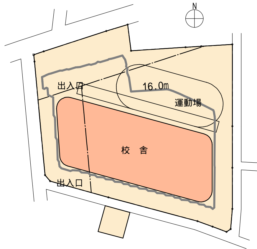
校舎を南側・運動場を北側へ配置した計画
