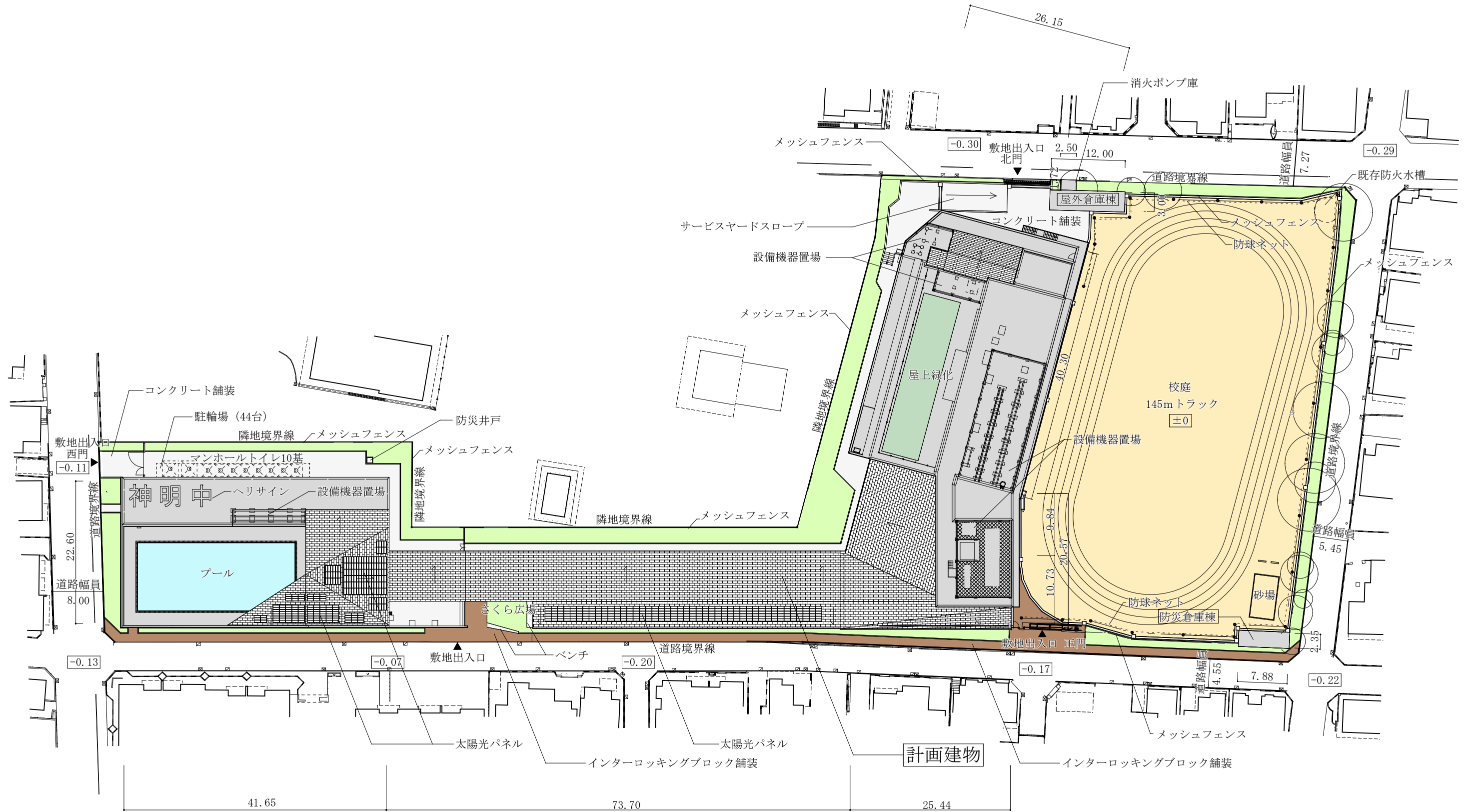
配置図
