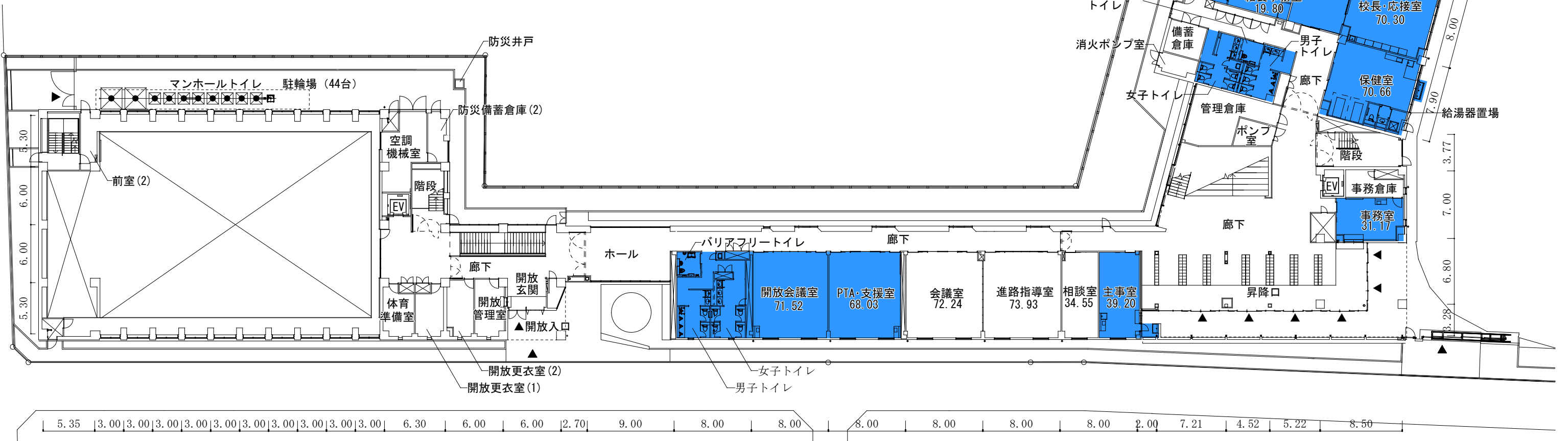
1階平面図
