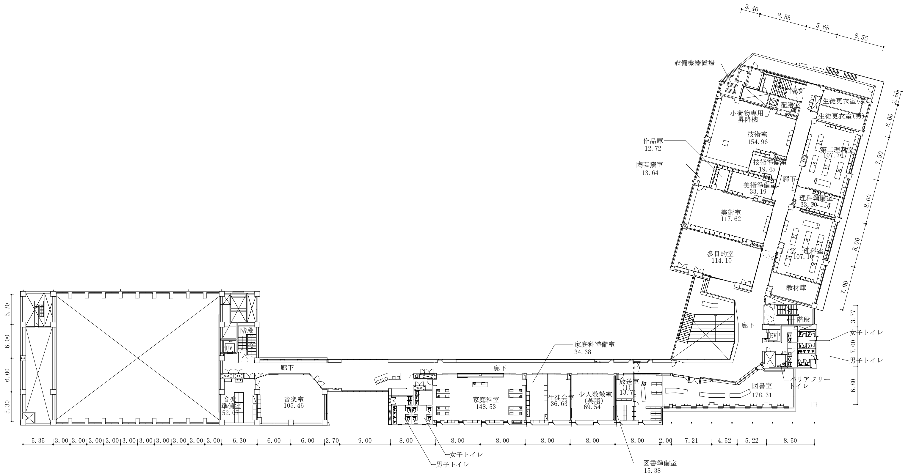
2階平面図
