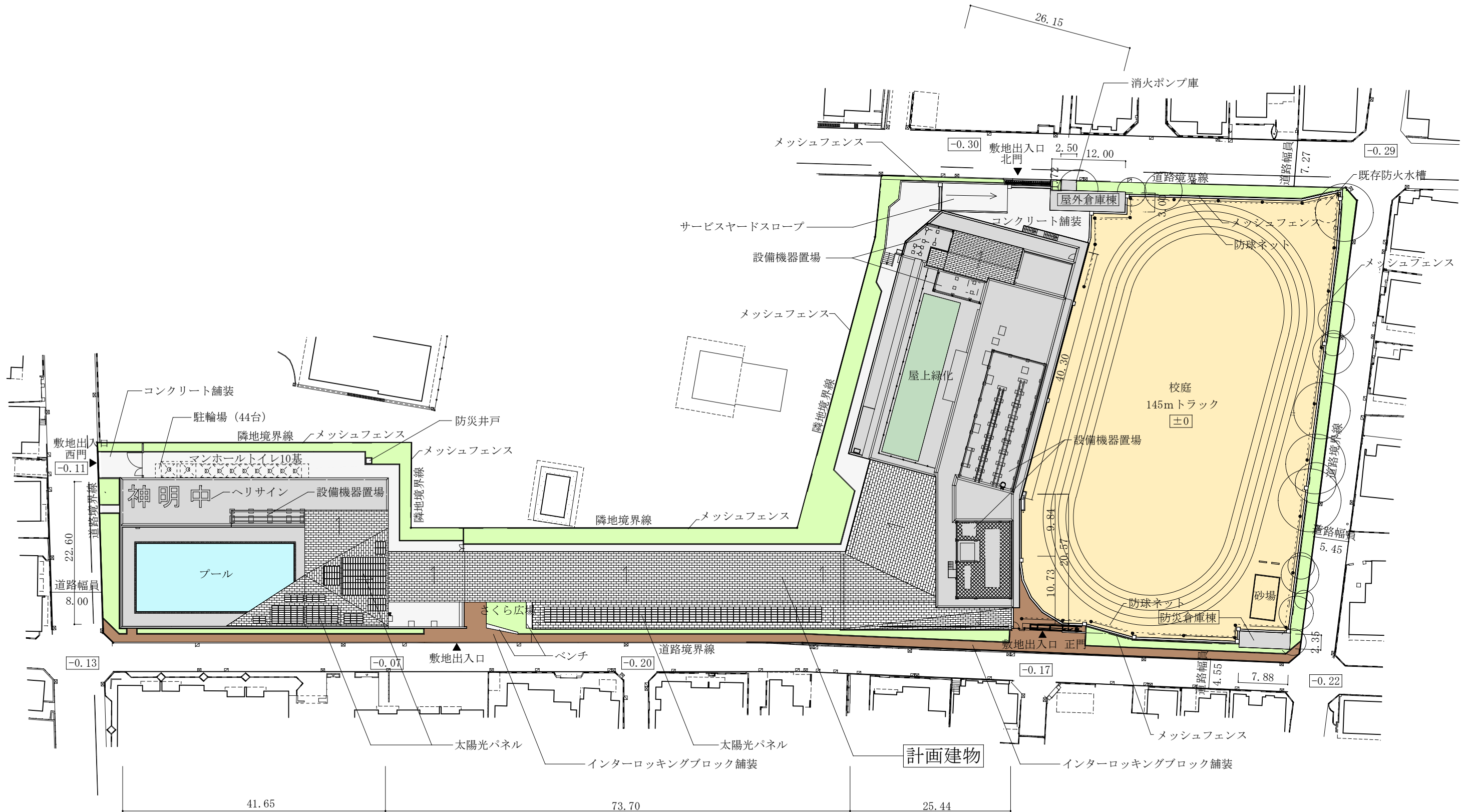
配置図
