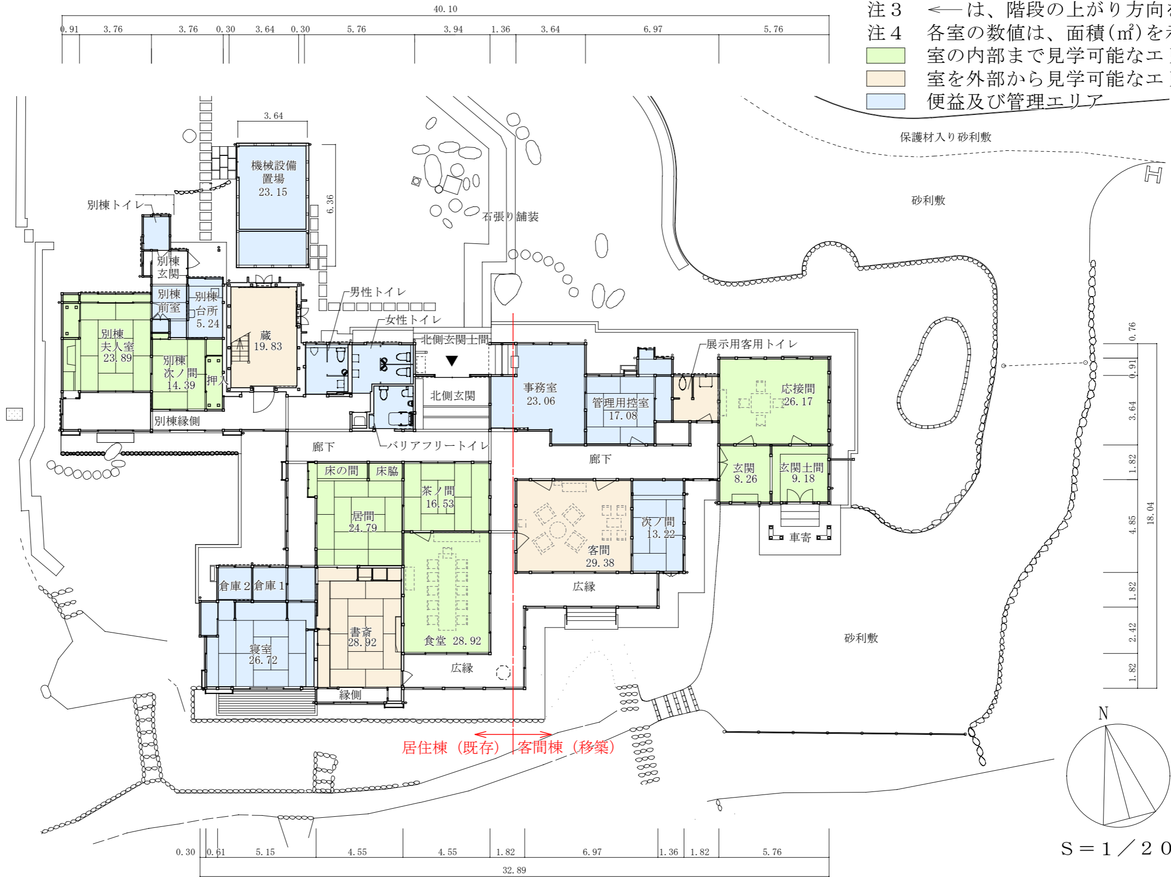
1階平面図
