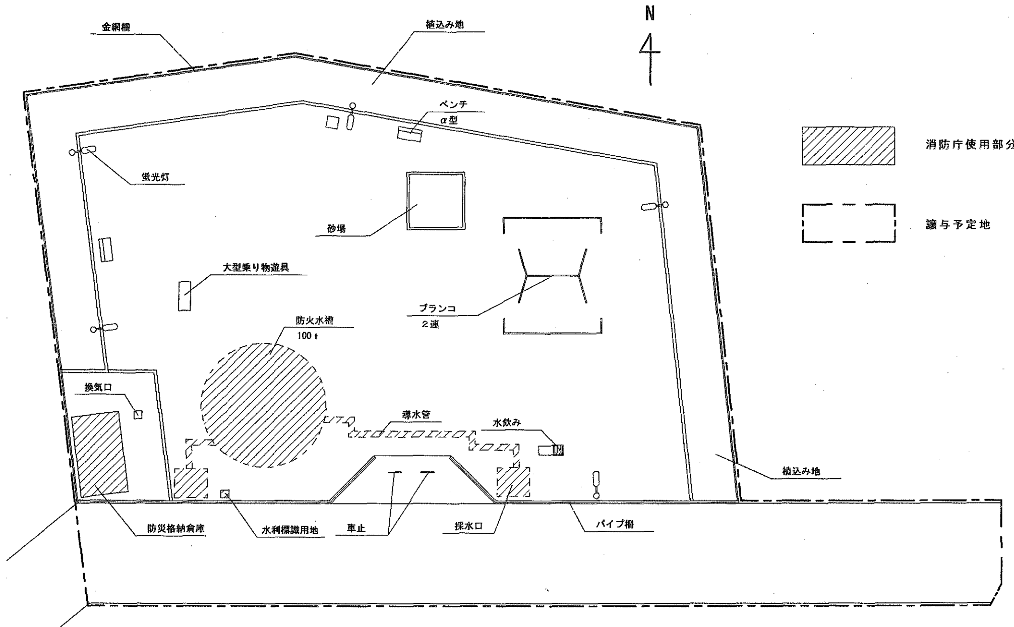
遊び場79番 平面図
