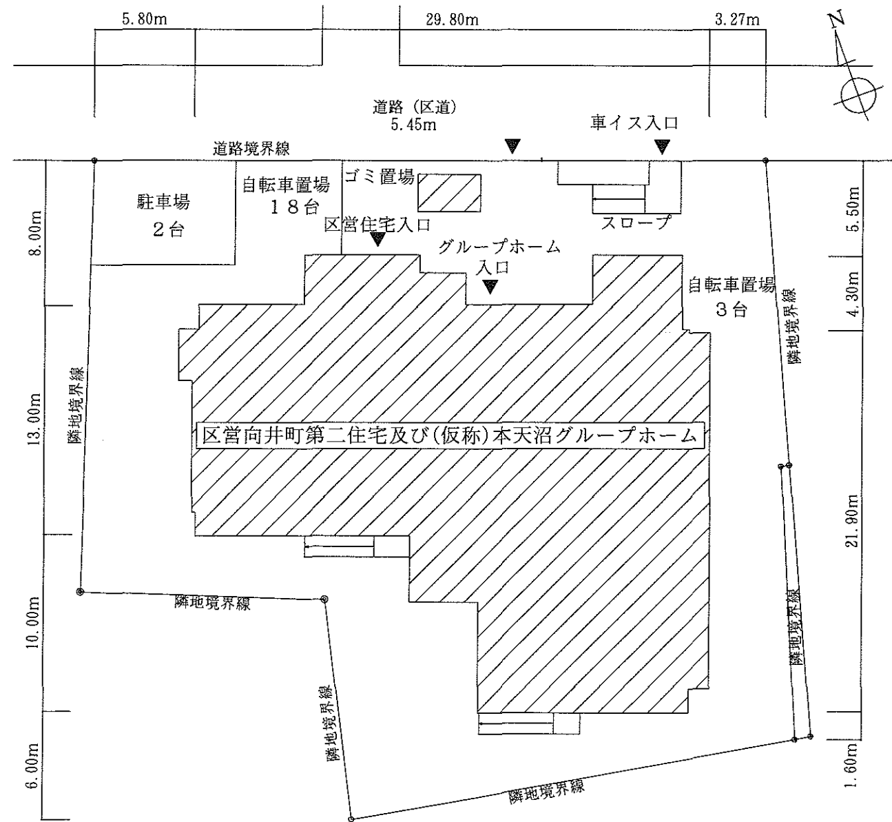
配置図 S=1/200
