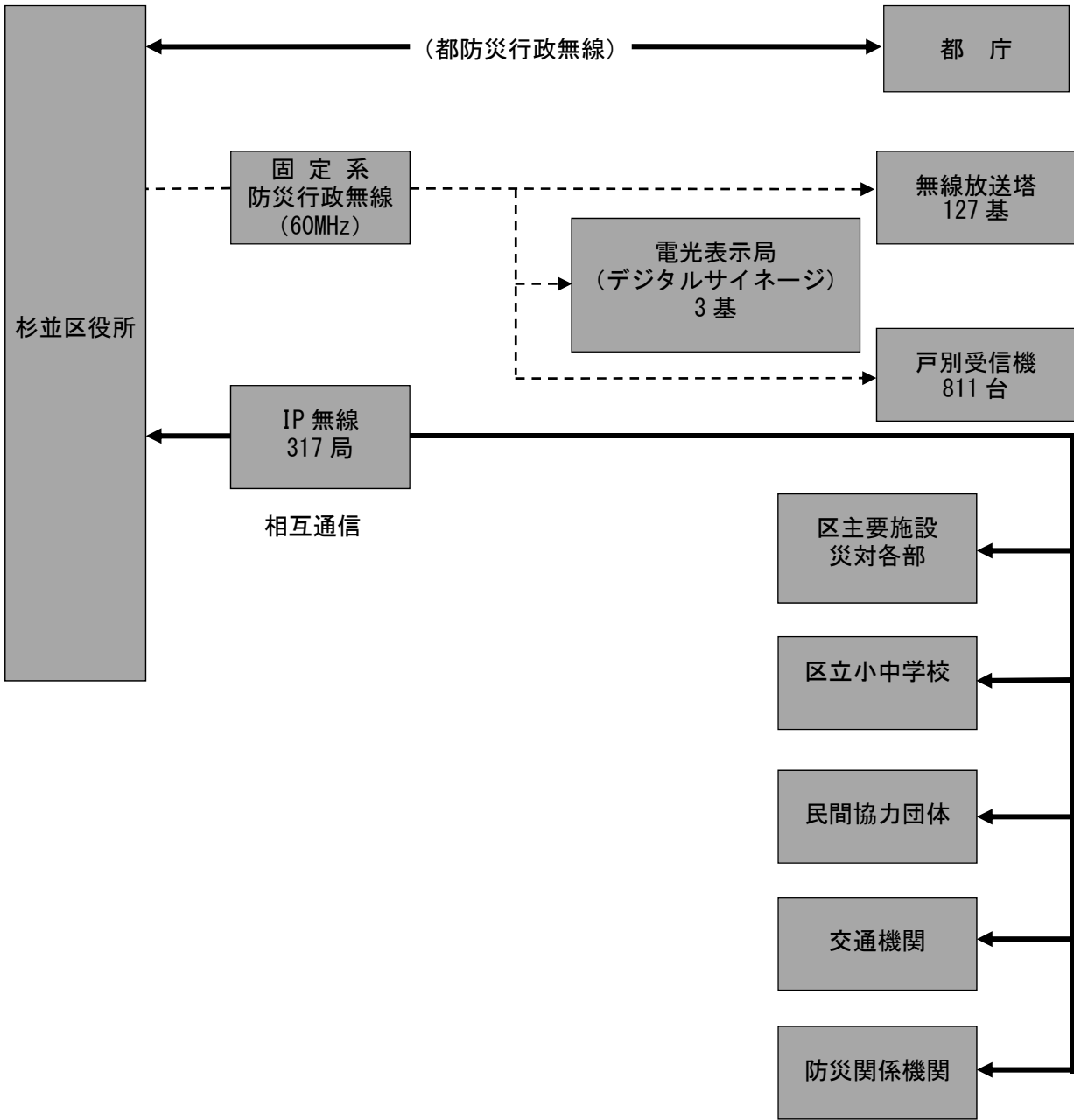
図表：杉並区防災行政無線系統図（令和5年(2023年)8月現在）
