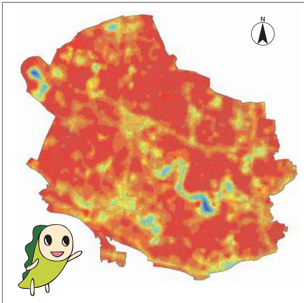
人工衛星のデータからみた杉並の都市熱状況(2023年7月27日)
