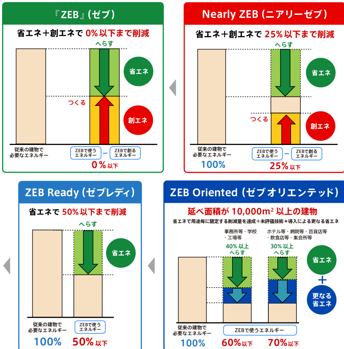
★図表 18 ZEB シリーズの概念図
