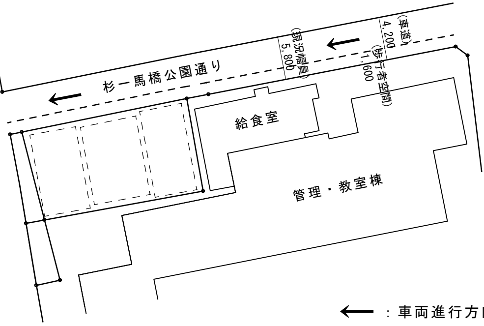
現況配置図 S=1/500
