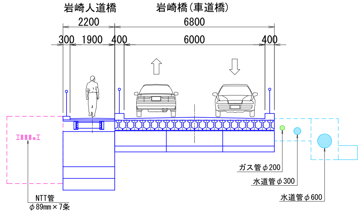
現況断面図
