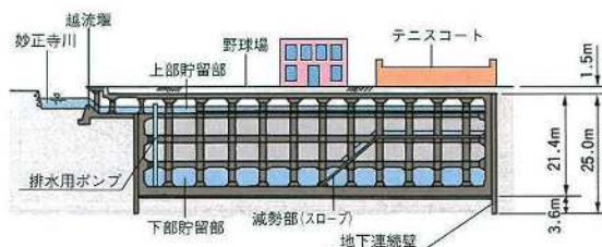
图 2-10 上高田調節池 断面図
