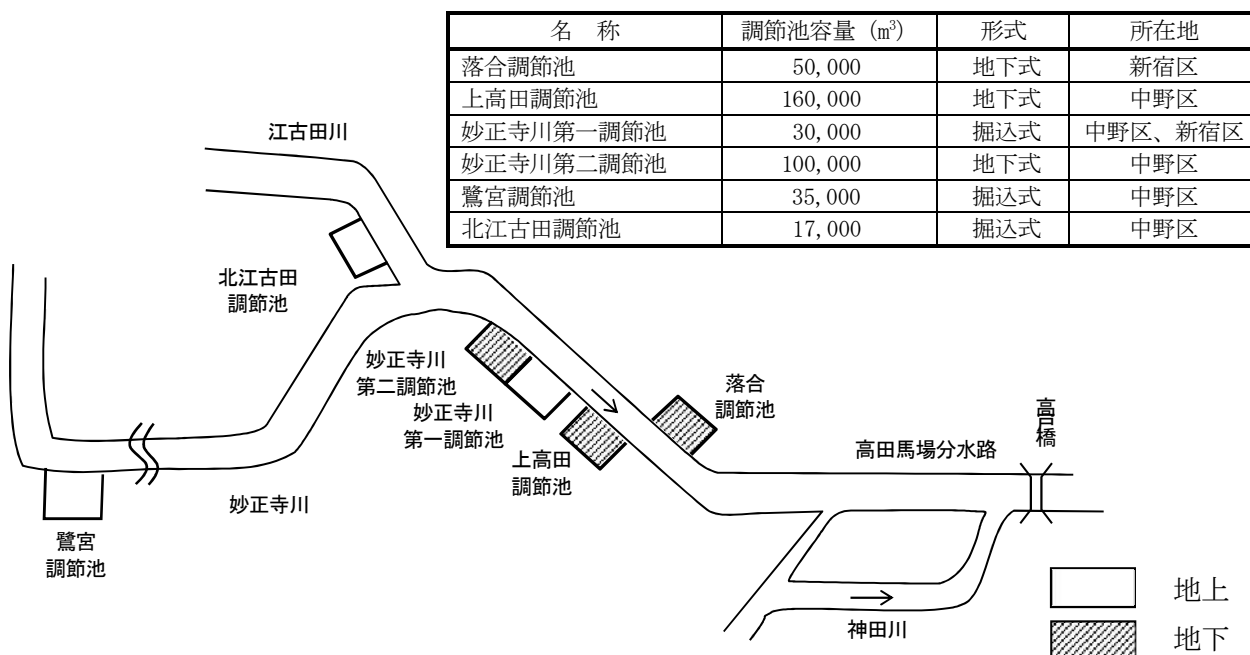
図 2-6 妙正寺川・江古田川の調節池
