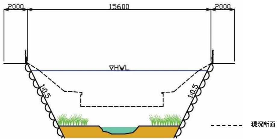
図4-2 標準断面図（善福寺川）
