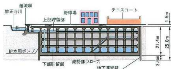
図 2-10 上高田調節池 断面図
