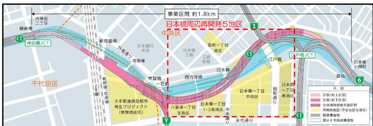
図4-12 首都高日本橋区間地下化事業及び日本橋周辺の市街地再開発事業位置図
