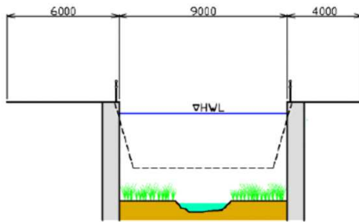
済美橋～松溪橋（和田堀公園・善福寺川緑地内）
