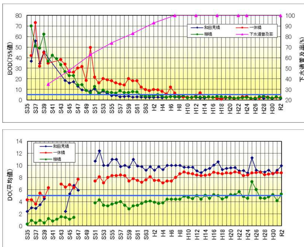
図2-14 神田川の水質の経年変化
