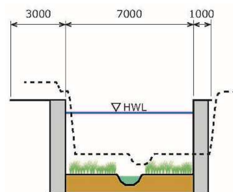
図4-4 標準断面図（江古田川）
