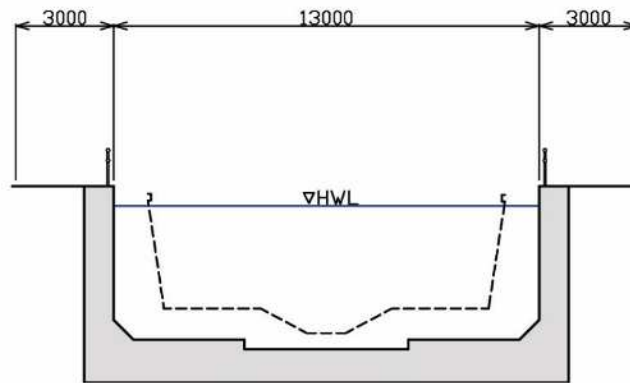
中野新橋～善福寺川合流点
