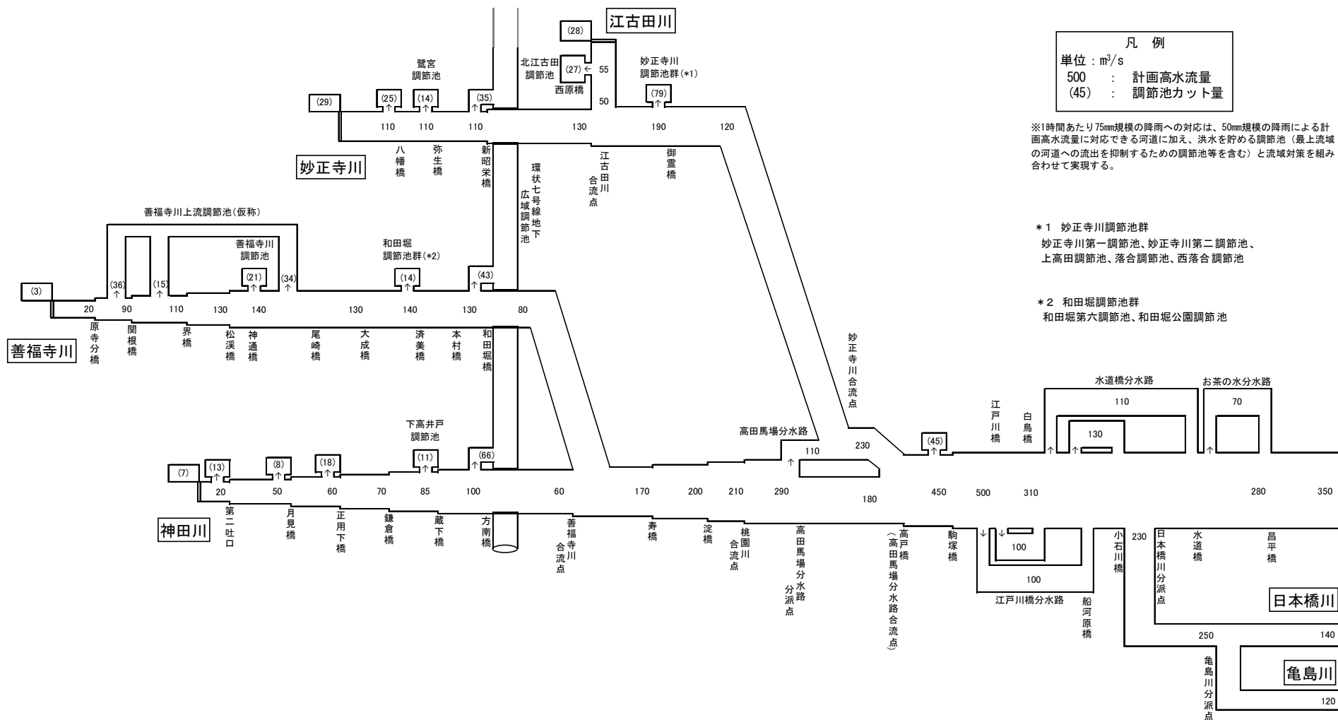
図 3-1 計画流量配分図
