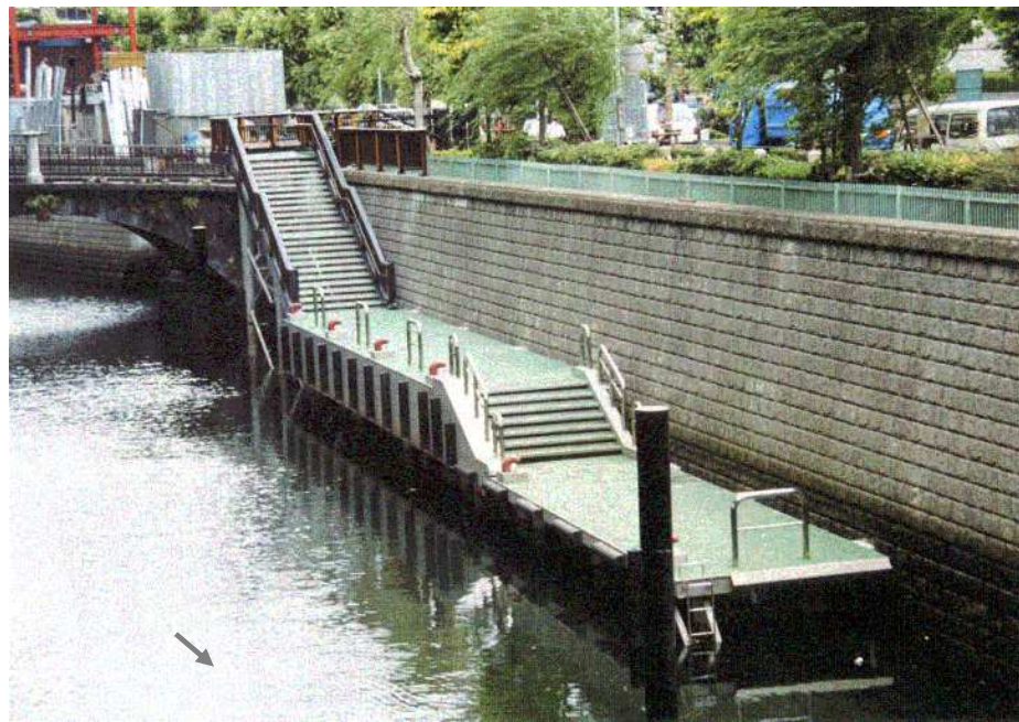
図 2－15 日本橋川 常盤橋防災船着場
