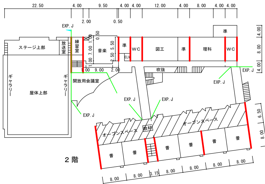
杉並第四小学校 各階平面図 S=1/800
