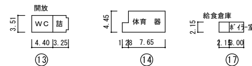
杉並第四小学校 各階平面図 S=1/800
