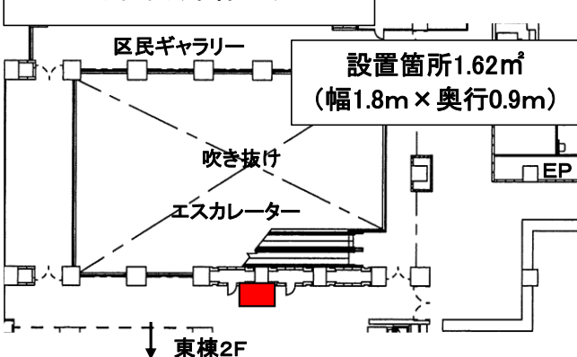
平面図(中棟2F)
