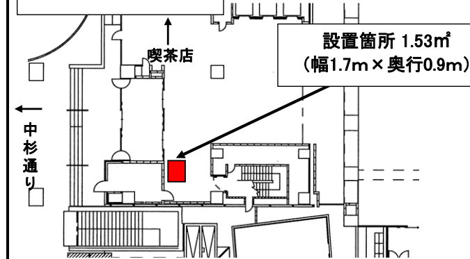
平面図(西棟1F)
