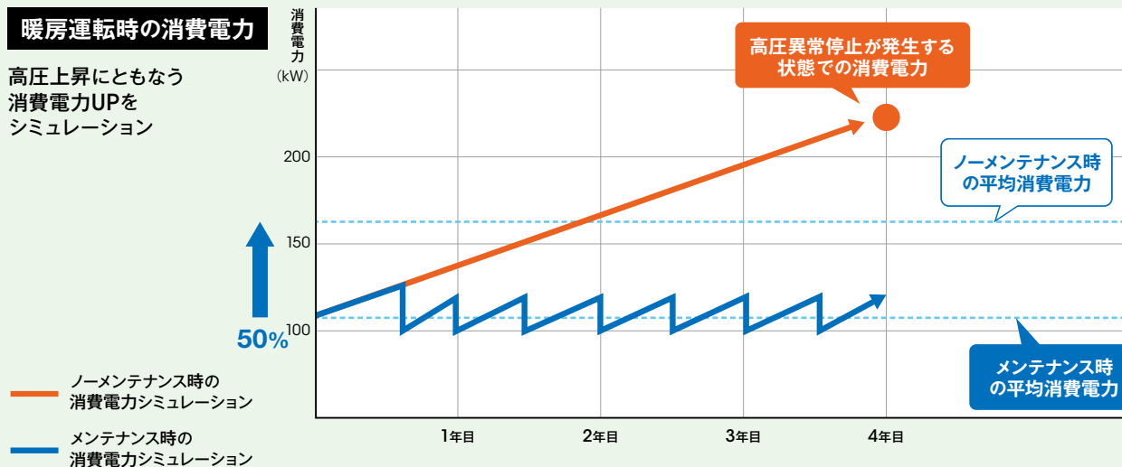
図Ⅲ-3-10 ノーメンテナンスによる消費電力の増加
