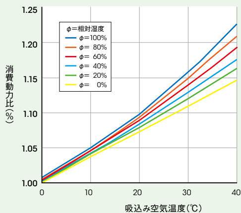
図Ⅲ-7-3 コンプレッサの吸込温度と消費動力の関係
