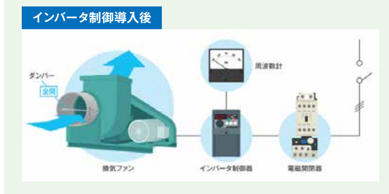
図Ⅲ-6-1 インバータ導入後の風量調整方法のイメージ
