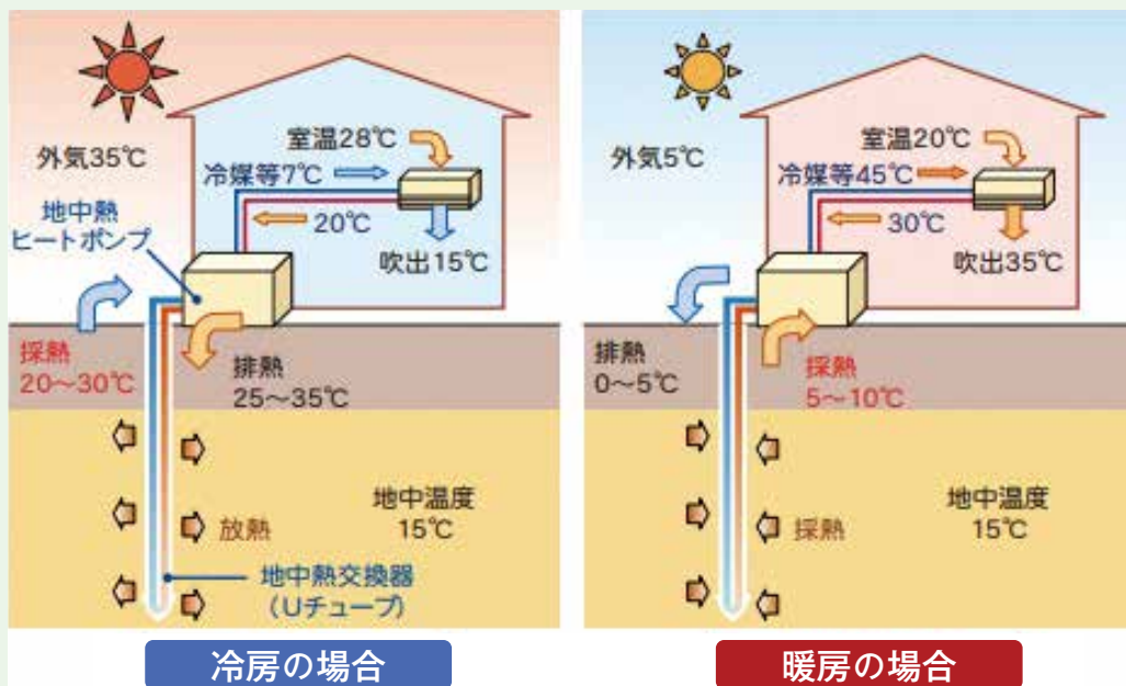
図IV-5-2 ヒートポンプシステムを活用した地中熱利用の例
