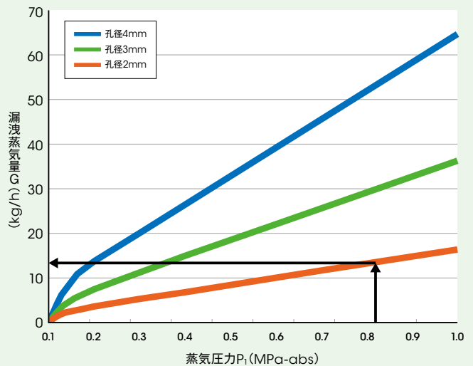
図III-8-7 小孔からの漏洩蒸気量
