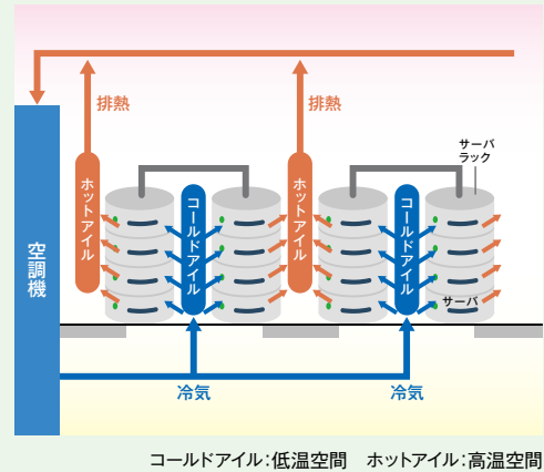
図Ⅲ-4-1 サーバ室空調システムの例
