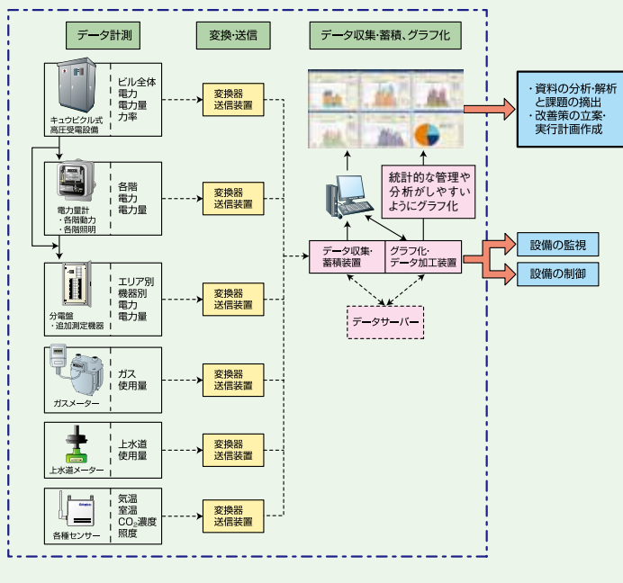
図Ⅲ-1-2 BEMSのイメージ
