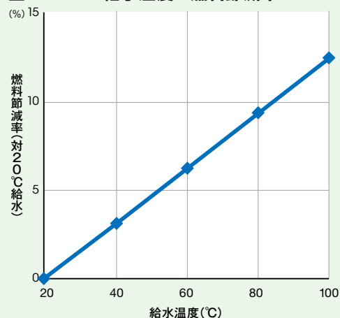
図Ⅲ-8-9 給水温度と燃料節減率
