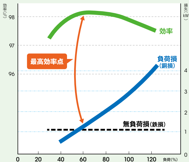
図Ⅲ-10-2 変圧器の効率特性
