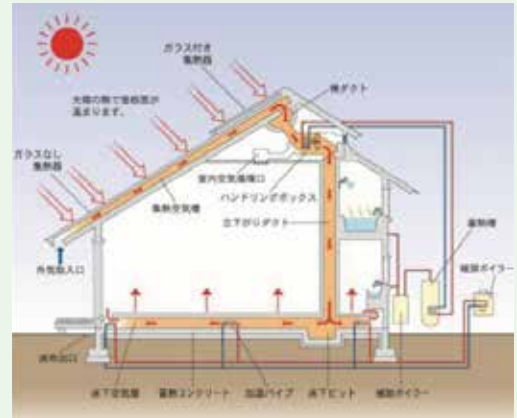
図IV-5-1 太陽熱利用システムのしくみ
