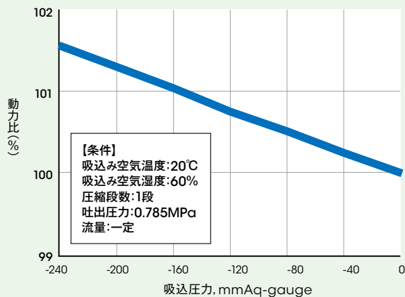
図Ⅲ-7-4 コンプレッサの吸込圧力と消費動力の関係
