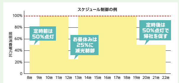
図Ⅲ-2-12 スケジュール制御の例
