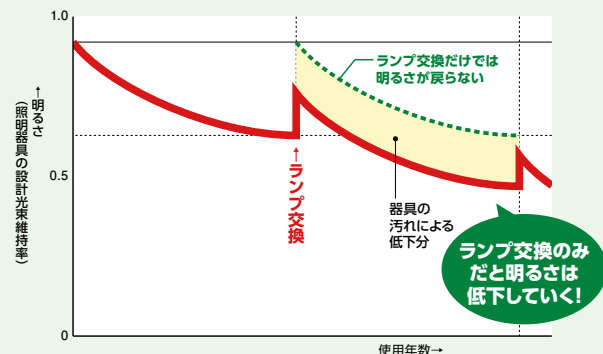
図Ⅲ-2-15 使用年数と明るさの変化イメージ
