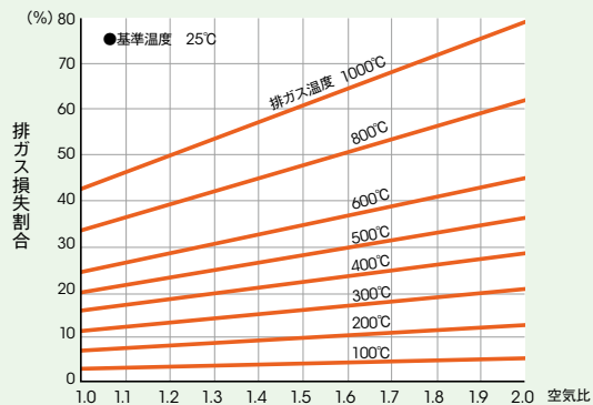
図Ⅲ-8-2 空気比と排ガス熱損失の関係
