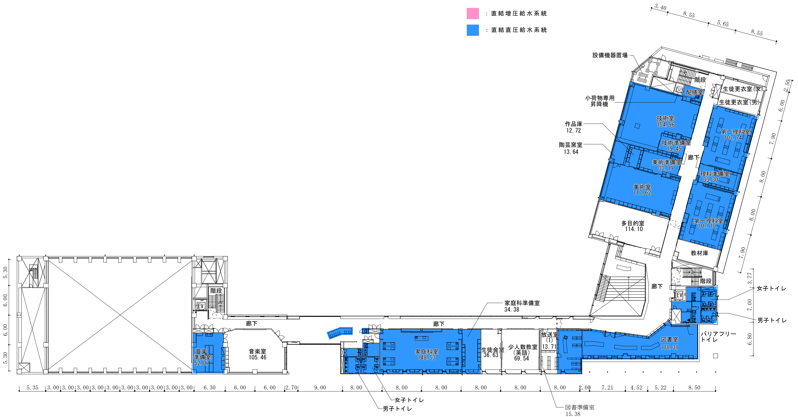
2階平面図
