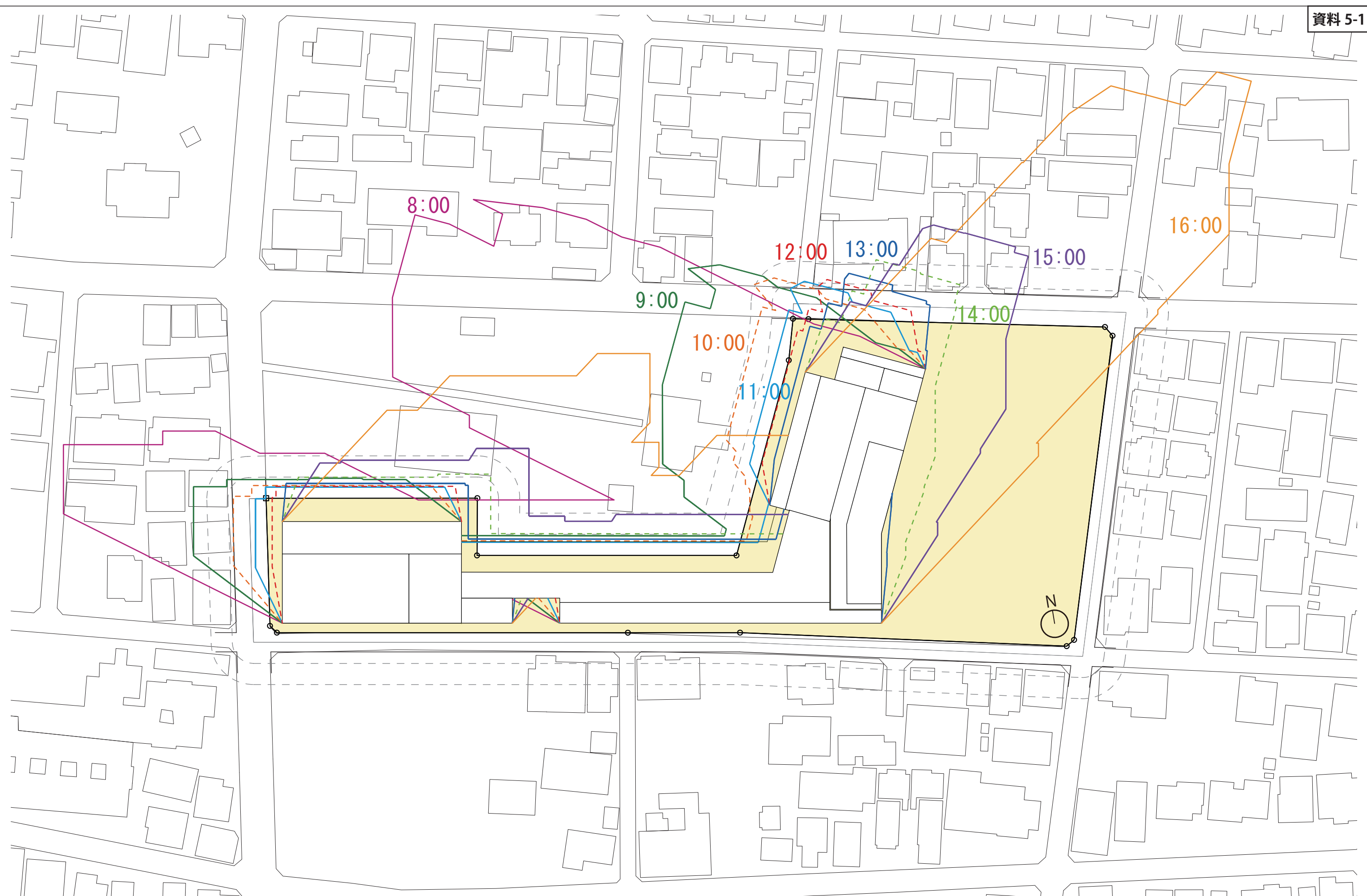
各時間日影図 冬至 受影面+1.5m
