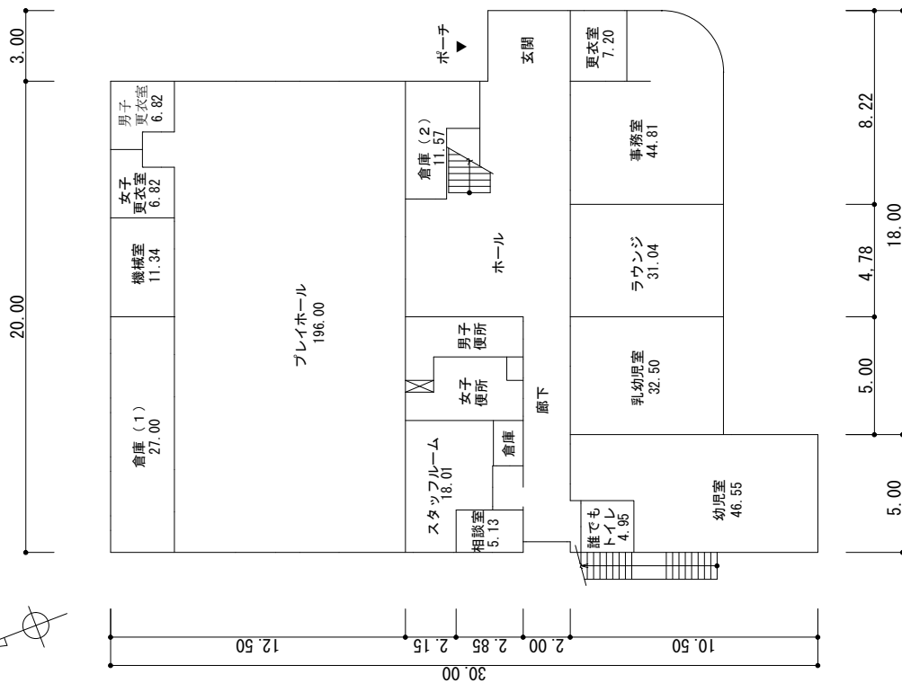
1階平面図 S = 1 / 300
