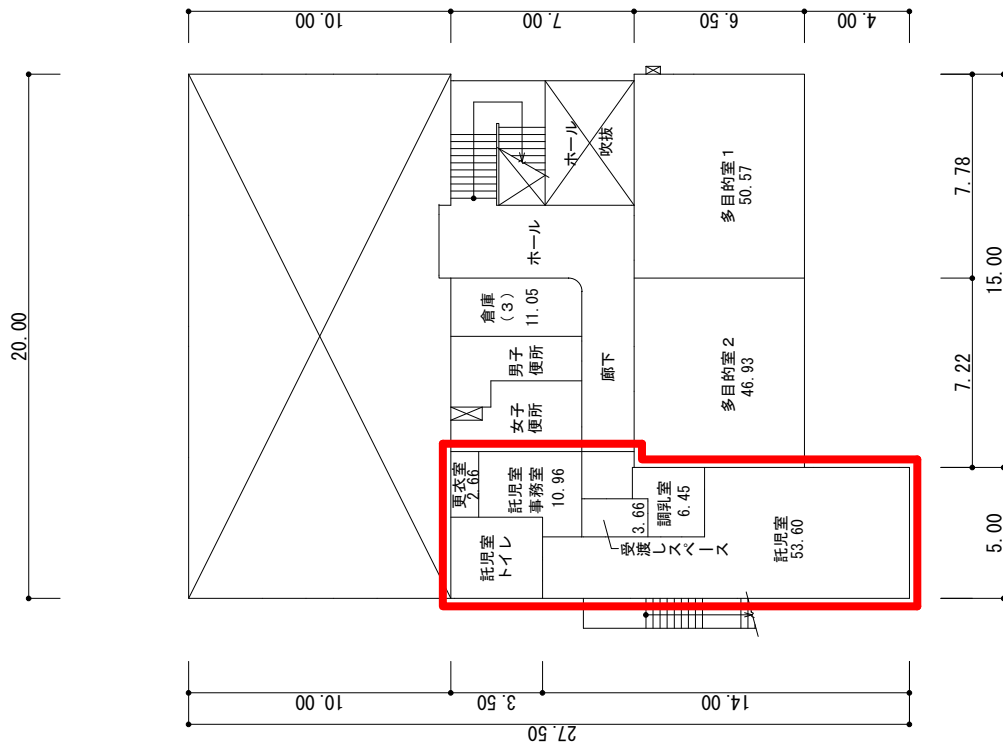
2階平面図 S = 1 / 300
