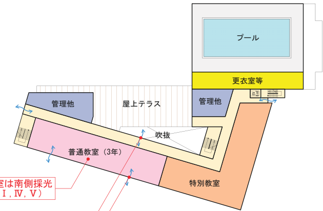
4階平面図
