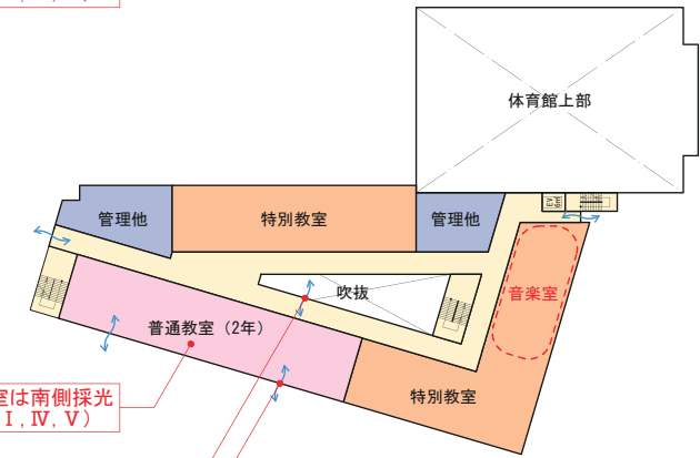
3階平面図
