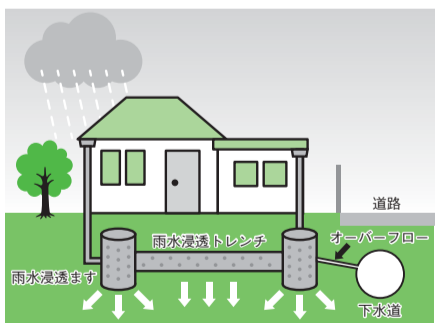
▲雨水浸透施設のイメージ
