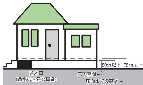
▲高床化のイメージ
