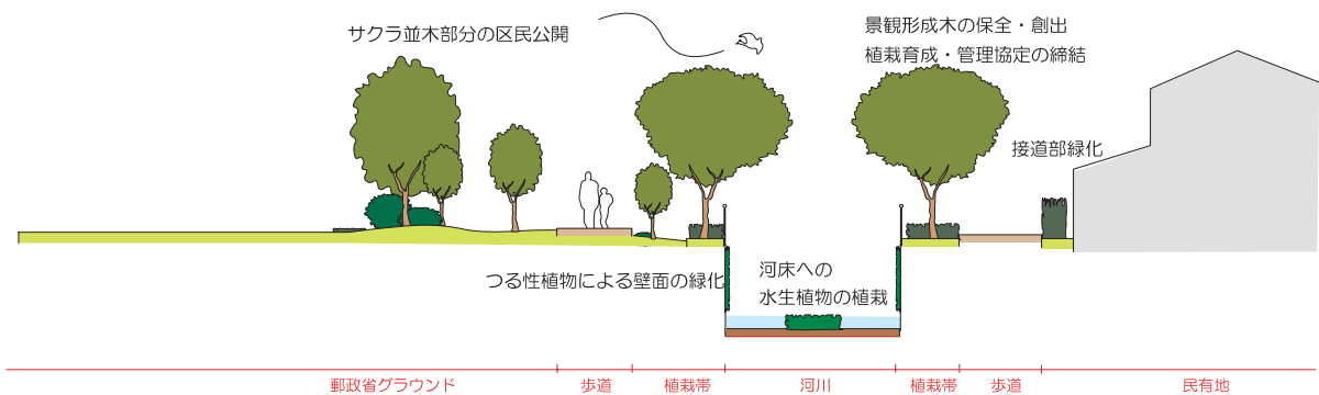
【断面図】
