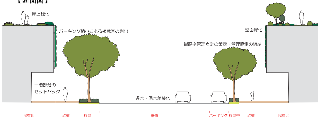
【断面図】
