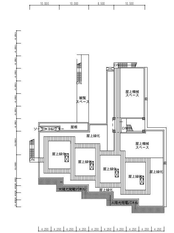
屋上階平面図
