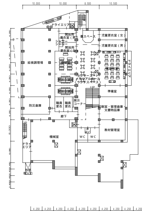
地下1階平面図
