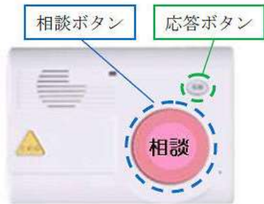
電源必要 AC100V 【相談ボタン付き通話器】 210(W) × 47(H) × 150(D) 電話機に接続
